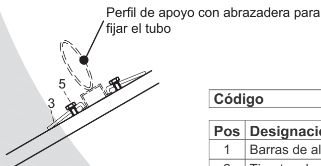
Fig. 1 Parte inferior
